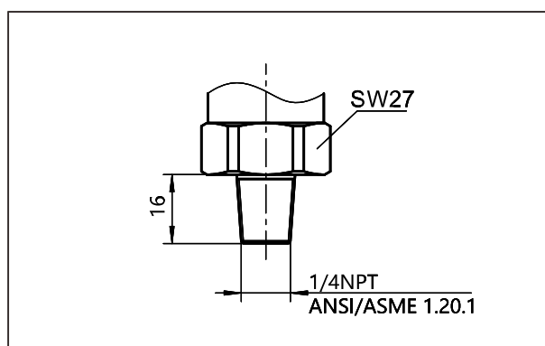
过程连接 (R02) (单位: mm)
