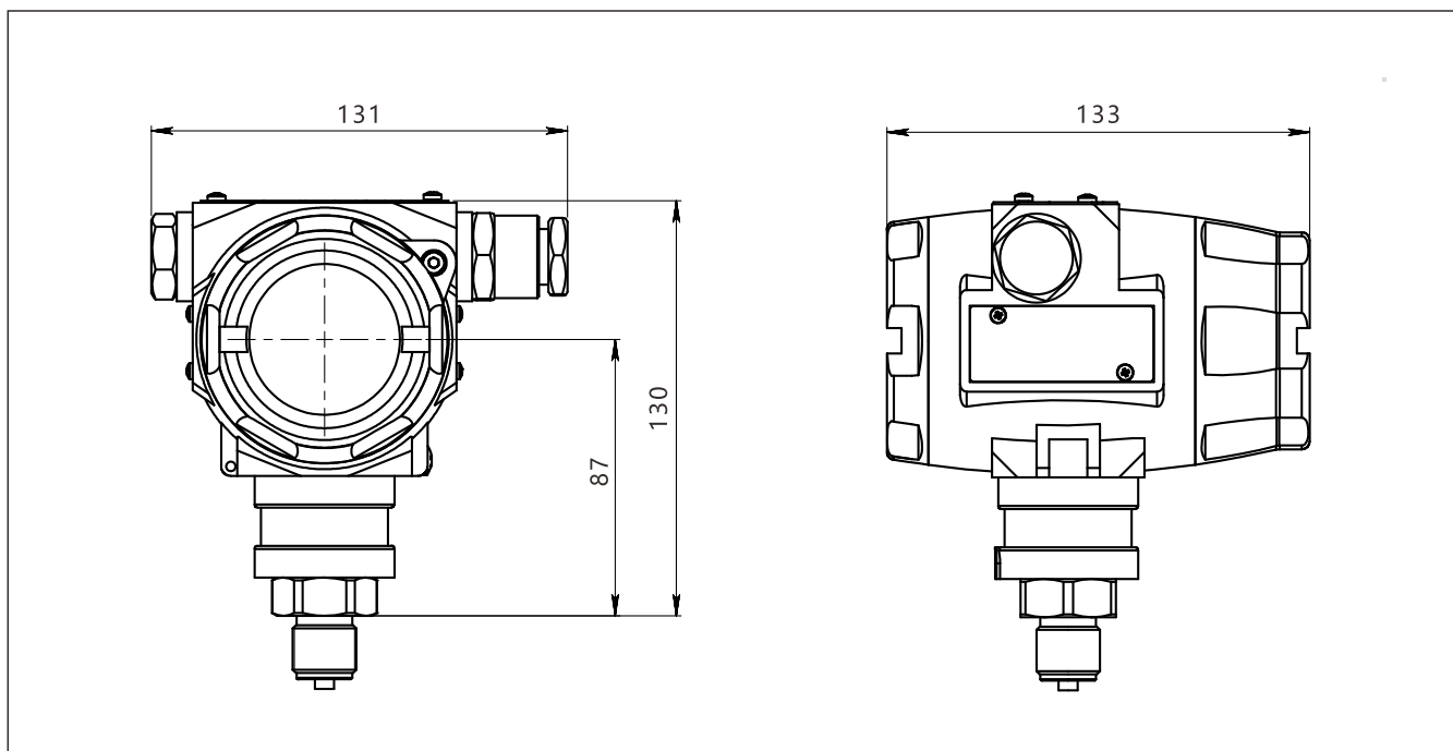
带显示 (C) 整机尺寸图 (单位: mm)
