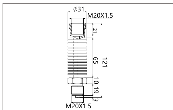
热交换连接件 (N2) (单位: mm)
