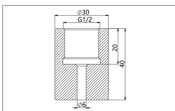
焊接转接件 (Z2) (单位: mm)
