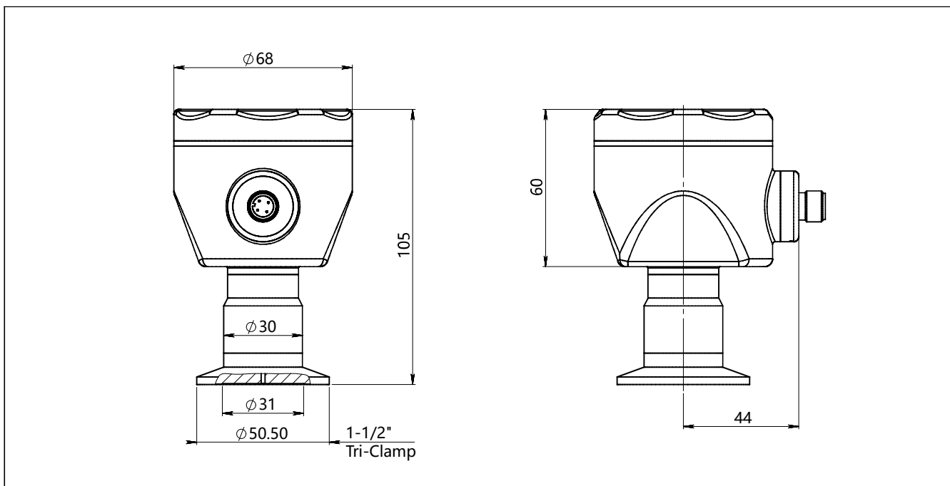
标准型带显示 (C) /不带显示 (A) 水平安装 (F2) 整机尺寸图 (单位: mm)
