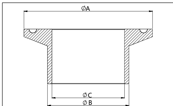
焊接转接件 (Z1-Z1) (单位: mm)
