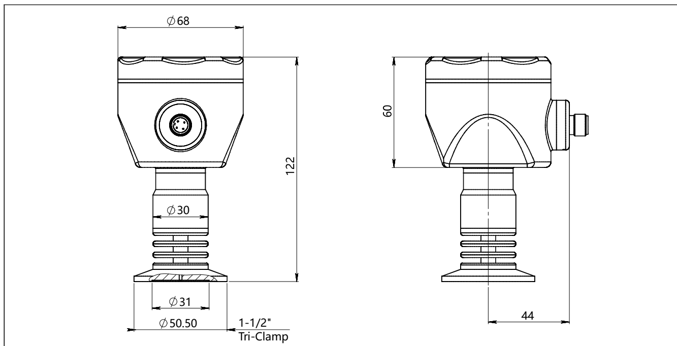
高温型带显示 (C) /不带显示 (A) 水平安装 (F2) 整机尺寸图 (单位: mm)
