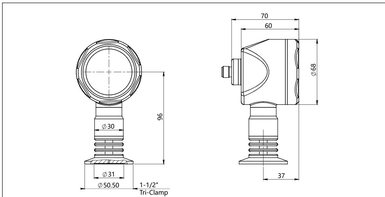
高温型带显示 (C) /不带显示 (A) 垂直安装 (F1) 整机尺寸图 (单位: mm)
