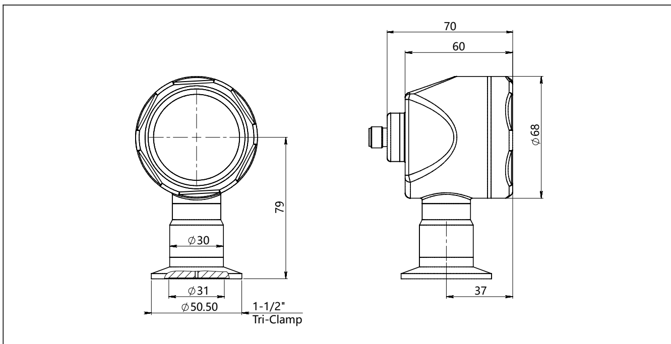
标准型带显示 (C) /不带显示 (A) 垂直安装 (F1) 整机尺寸图 (单位: mm)
